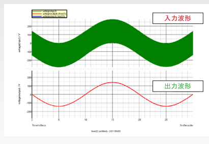
Fig.2 Fig.1のフィルター特性を有するインライン・パワーフィルターを回路シミュレートし、AC100V/50Hz電源波形にAC100V/10MHzのノイズ波形を重畳した波形を入力し、高周波ノイズ遮断効果をシミュレート。
